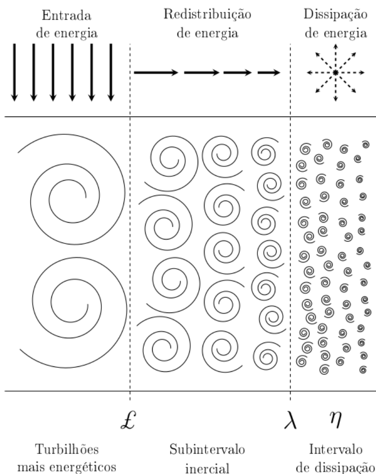
Figura 1 – Representação da cascata de energia cinética turbulenta. Adaptada de Puhales et al. (2015).
