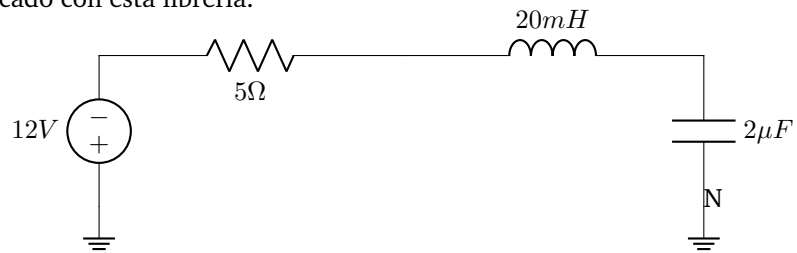
Figura 3.5: Ejemplo del uso de la libreria circuitikz
