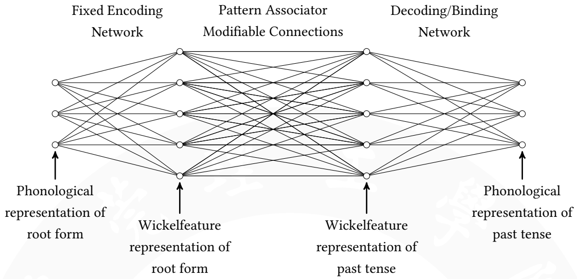
图 3-3 神经网络示意图
