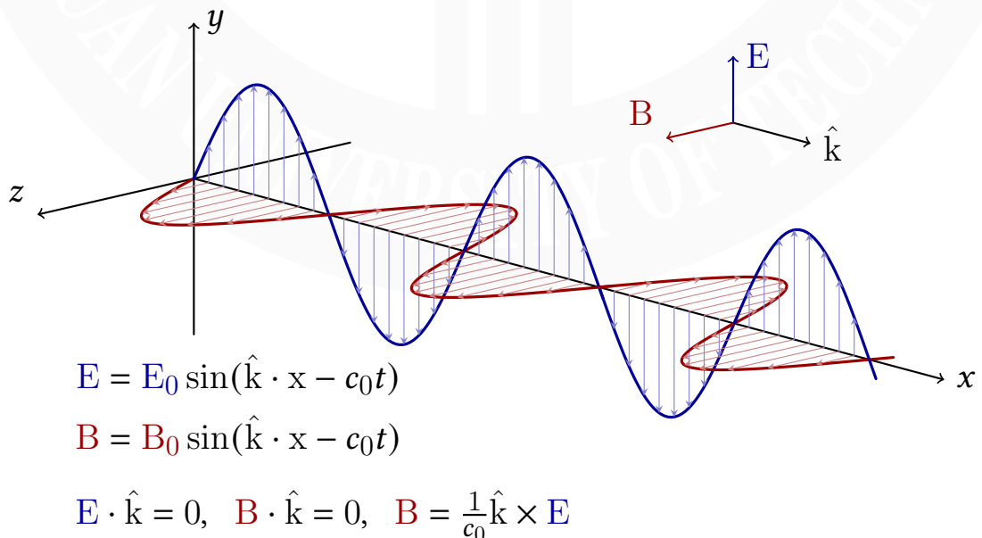
图 3-8 电磁波示意图
