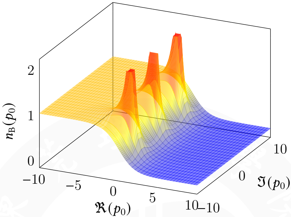
图 3-6 玻色爱因斯坦分布示意图
